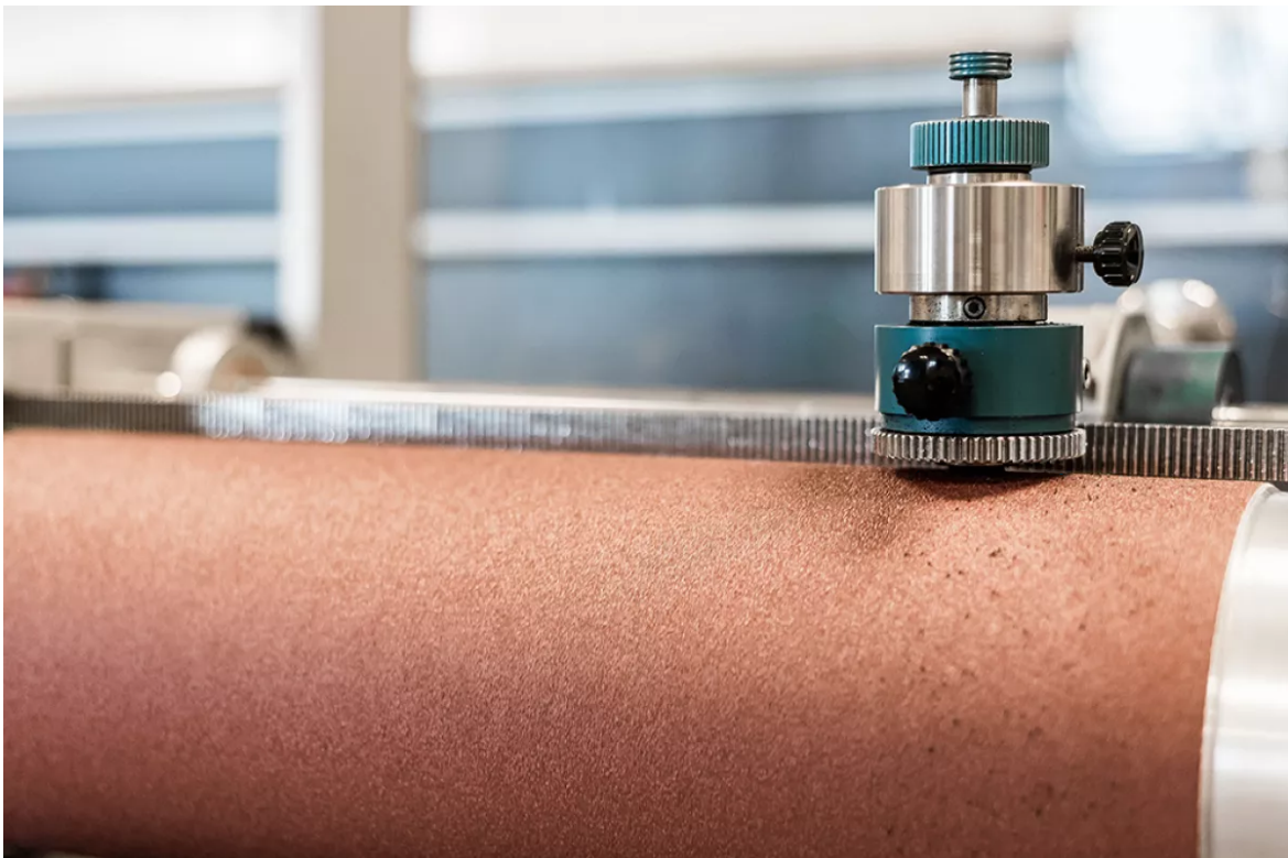
ISO 4649 / DIN 53516 abrasion testing
