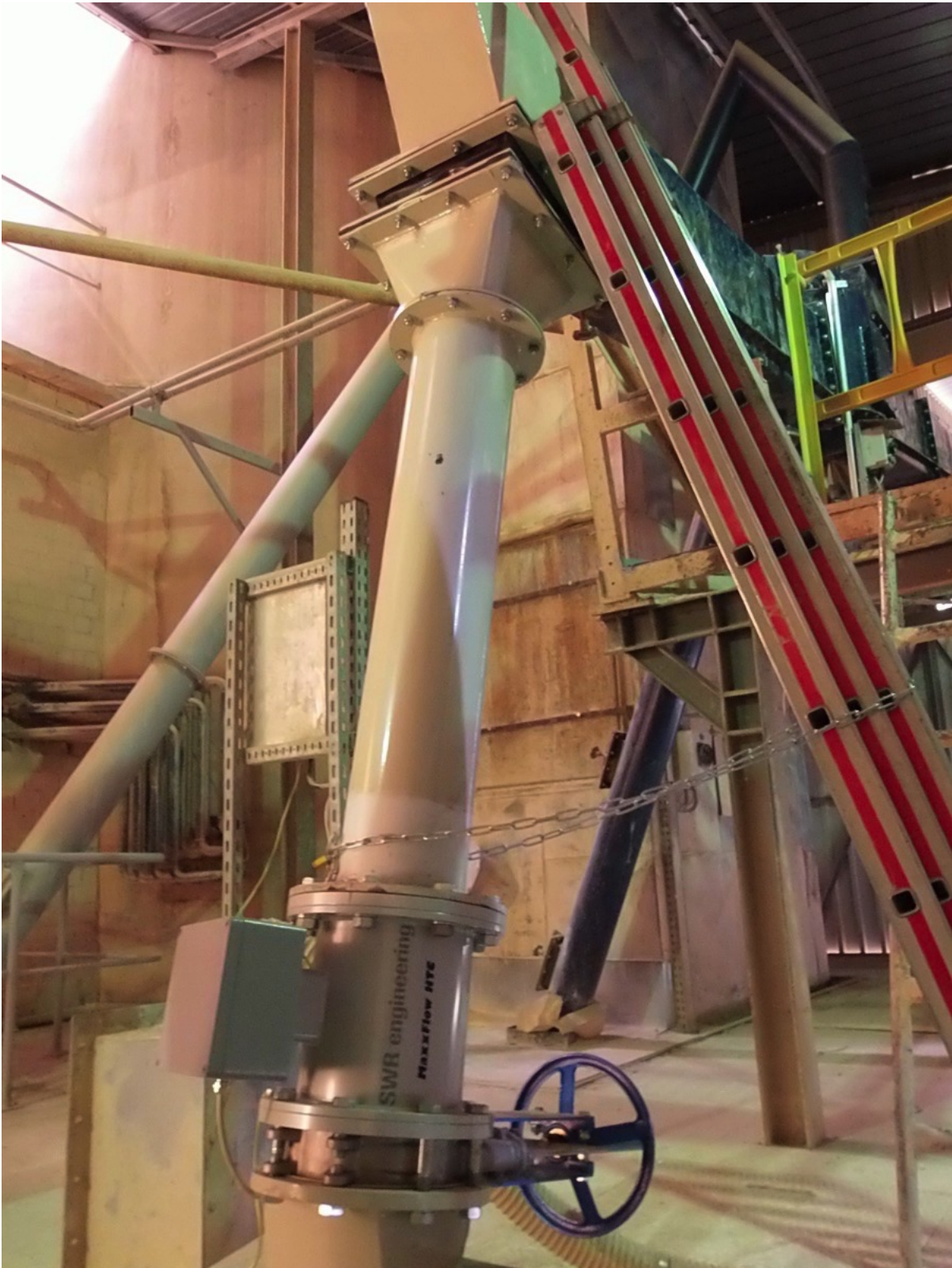
Mühlenrücklaufmessung mittels MaxxFlow in der Zementindustrie. (Bild: SWR engineering)
